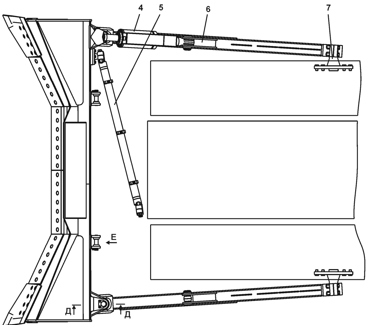
Рисунок 8.16 Оборудование бульдозерное сферическое Figure 8.16 Dozer spherical equipment
