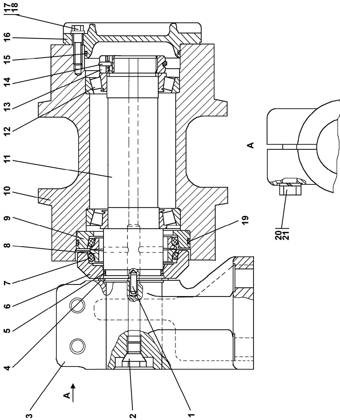
Рисунок 8.12 Каток поддерживающий Figure 8.12 Support roller
