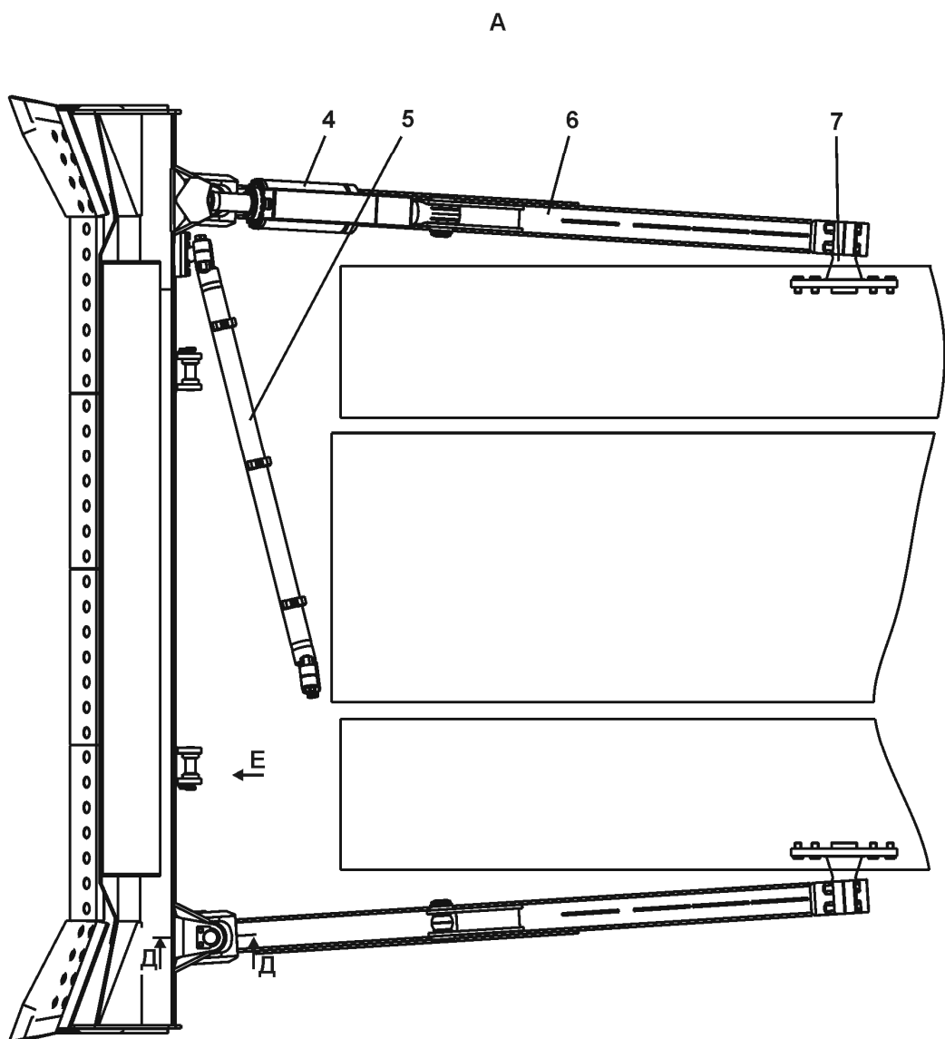
Рисунок 8.18 Оборудование бульдозерное полусферическое Figure 8.18 Dozer hemispherical equipment
