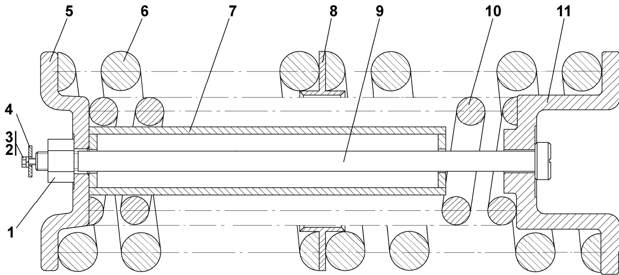
Рисунок 8.14 Механизм сдвигания Figure 8.14 Track-release mechanism
