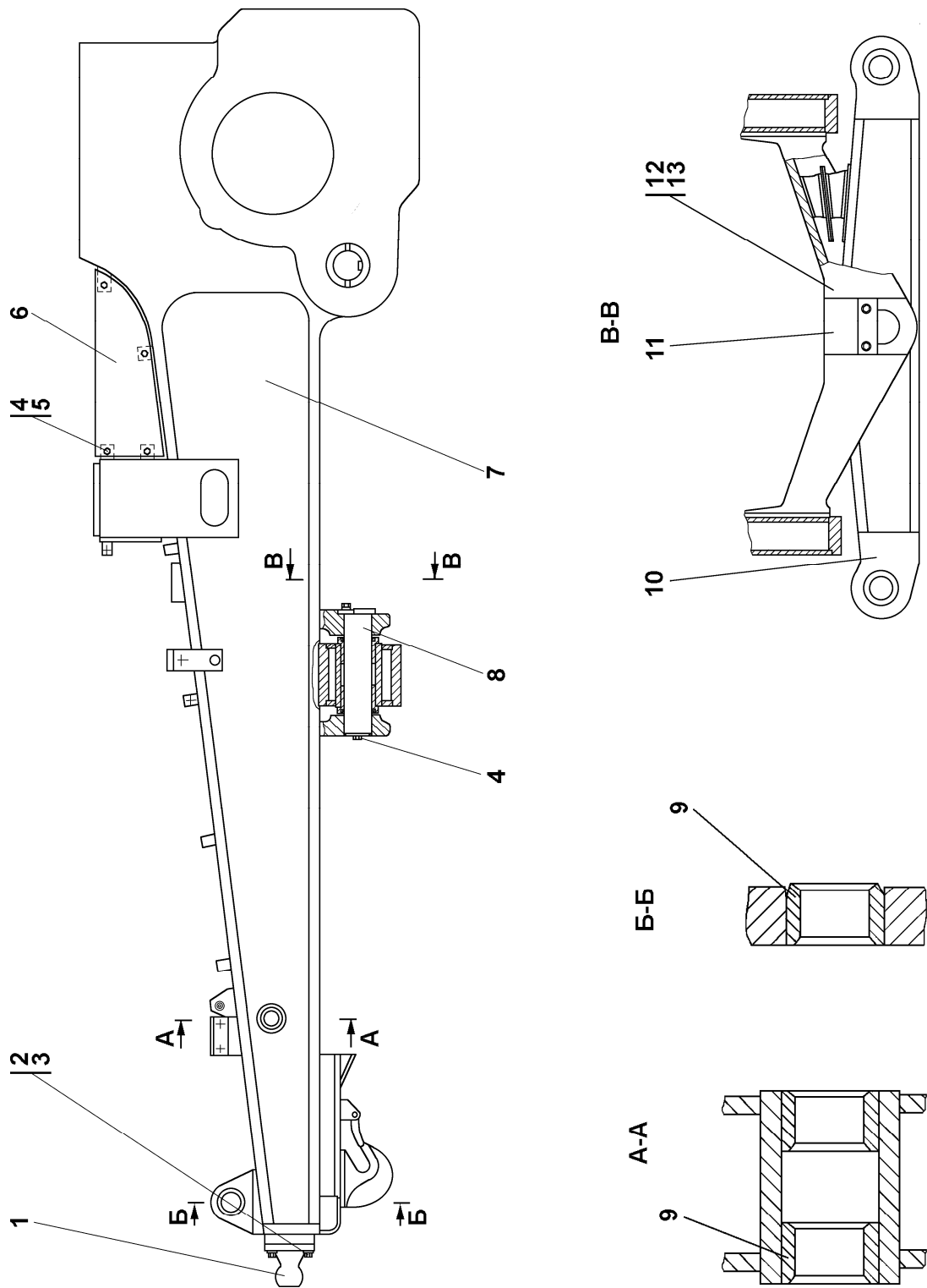
Рисунок 8.5 Рама Figure 8.5 Frame
