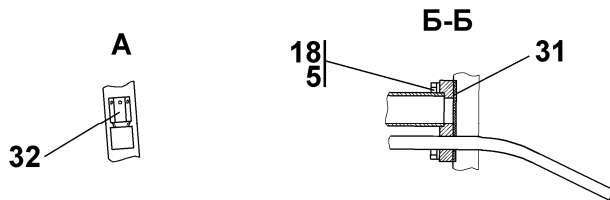
Рисунок 8.1 Установка трансмиссии Figure 8.1 Transmission mounting
