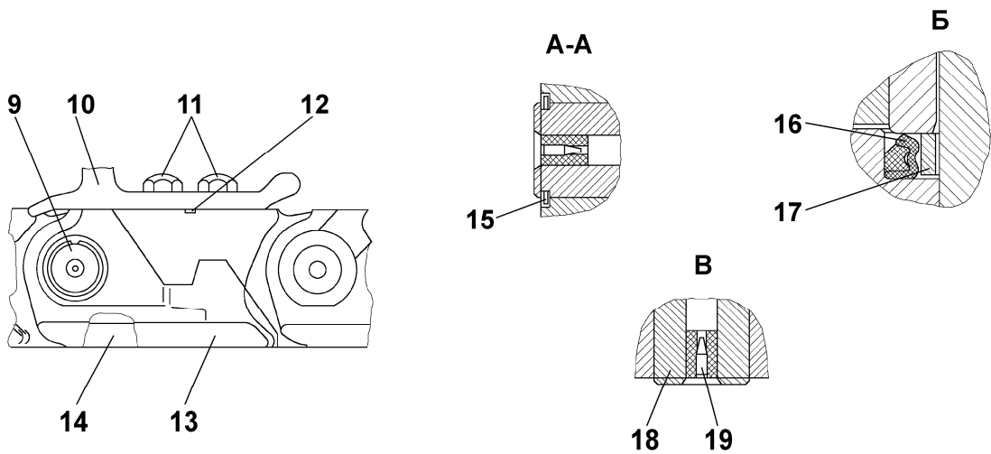
Рисунок 8.11 Гусеница Figure 8.11 Track
